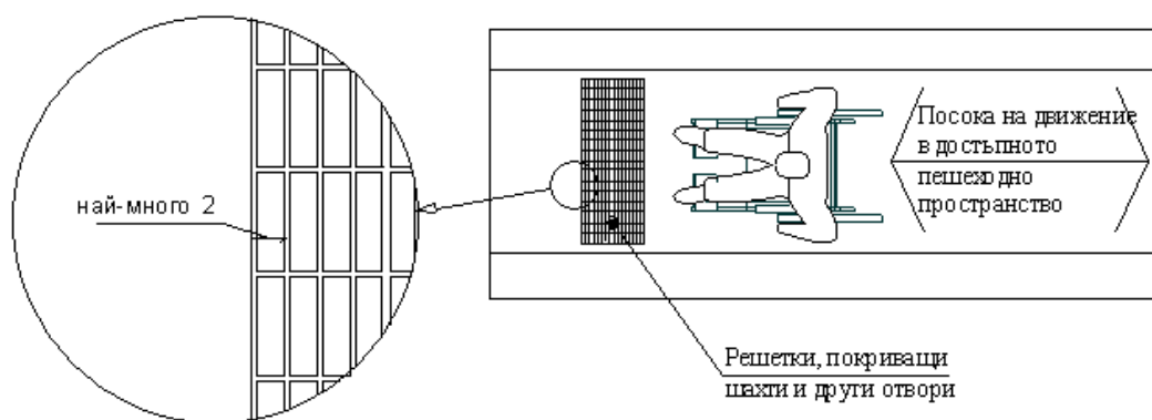
Фиг. 8. Ориентация на решетките, покриващи шахти и други отвори (размерите са в см)
