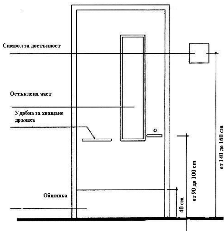
Фиг. 32. Достъпни врати по достъпните маршрути
