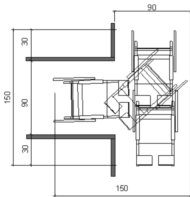
Необходима площ за завъртане на инвалидна количка на 180°
