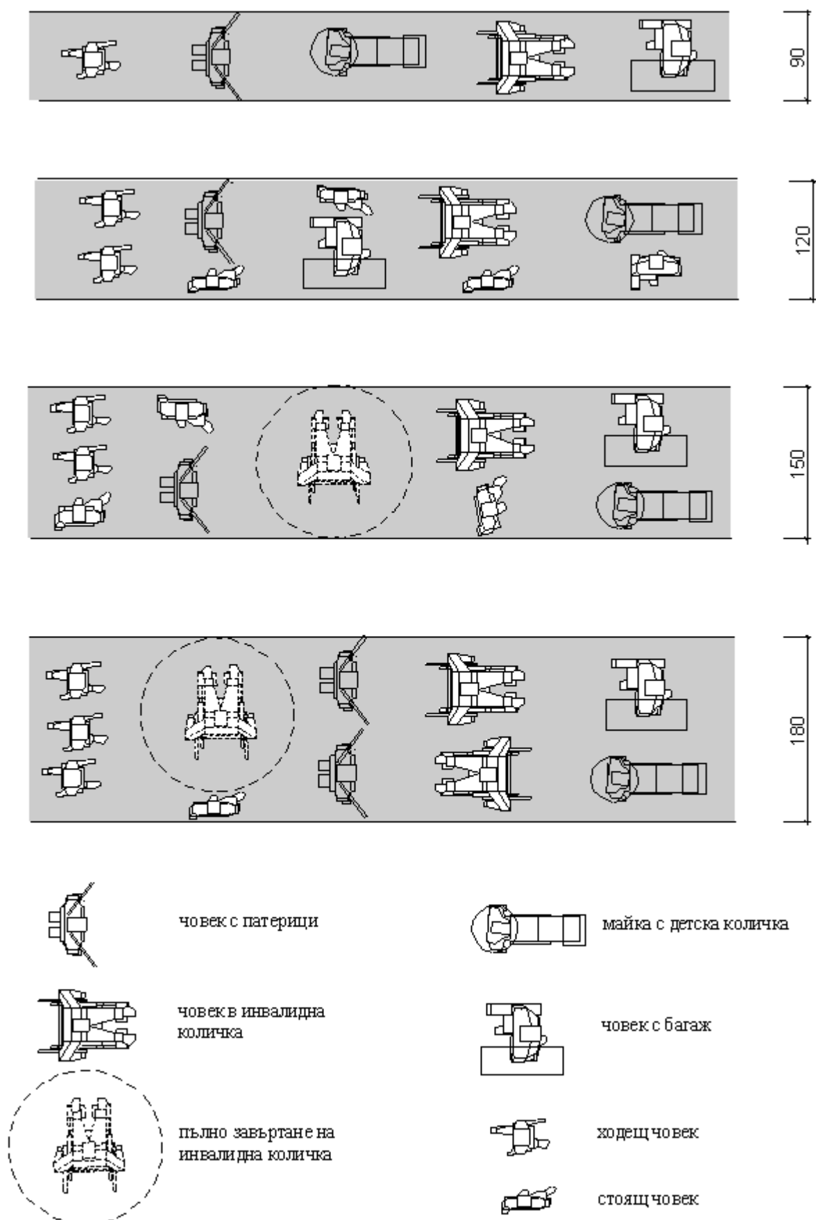
Фиг. 4. Минимална широчина на достъпните марирути
